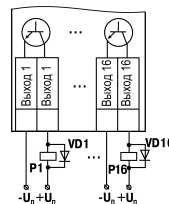
Рисунок 4 – Схема подключения нагрузок к ВЭ типа «К»
